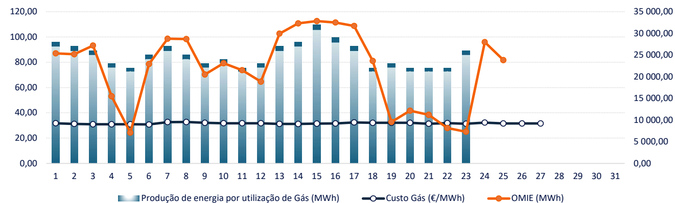
Custo Grossista Energia (€/MWh) Vs Custo Gás (€/MWh) Vs Prod. Energia por Gás (MWh)
